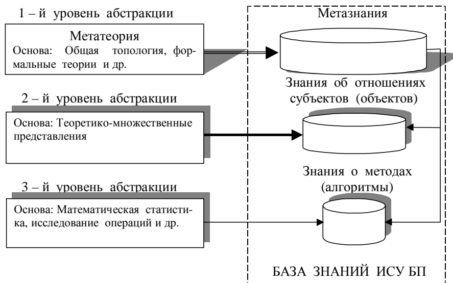
Рис. 1. Схема соответствия форм познания сложной системы (уровни абстракции), уровням иерархии их представления в базе знаний интеллектуальной системы
